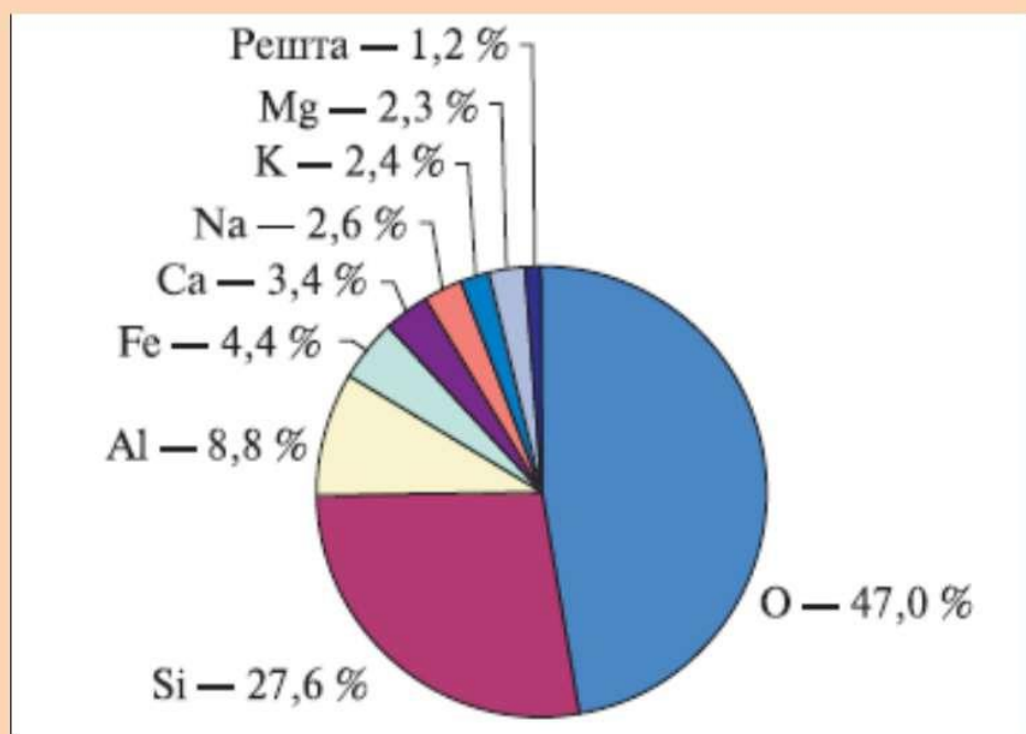
Вміст хімічних елементів у земній корі
